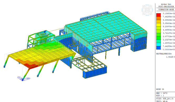
Primo modo di vibrare dell'immobile
