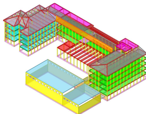
Modello ad elementi finiti dell'Istituto Percoto
