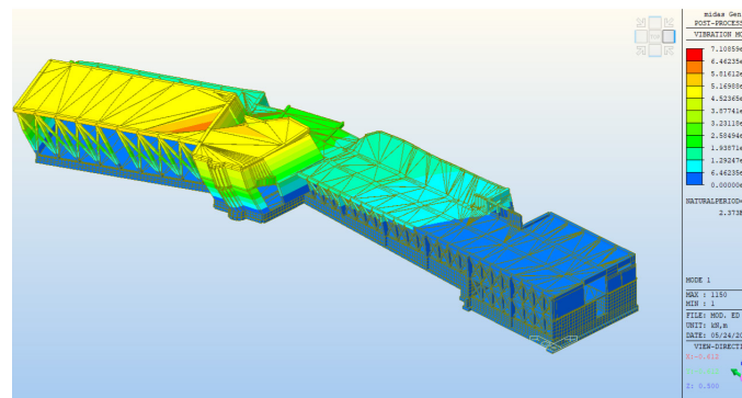
Principale modo di vibrare dell'immobile
