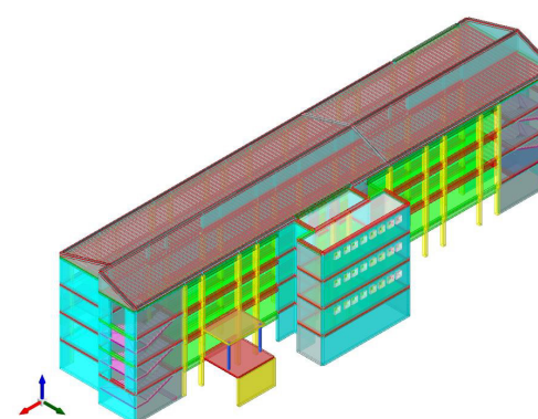
Modello ad elementi finiti del Liceo Marinelli
