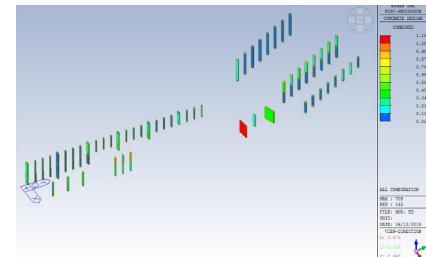
Verifiche strutturali sugli elementi portanti verticali
