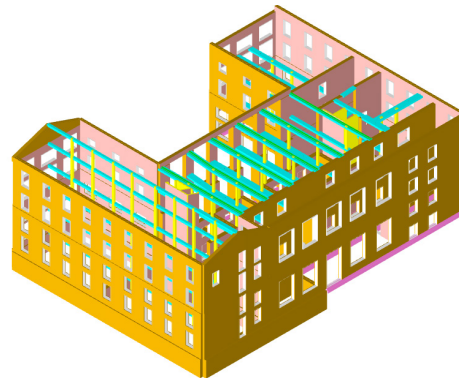
Modello FEM dell'immobile - ala storica
