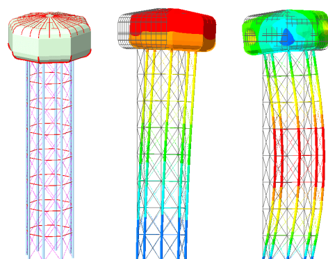
Modello FEM e principali modi di vibrare ella torre piezometrica
