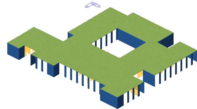
Modello FEM dell'immobile
