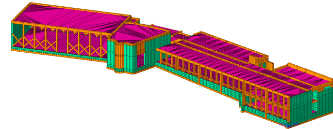
Modello FEM dell'immobile
