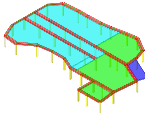
Modello ad elementi finiti del complesso scolastico
