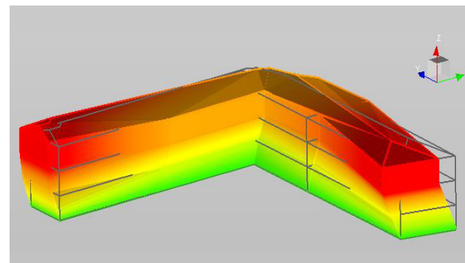
Modo di vibrare individuato tramite prova dinamica
