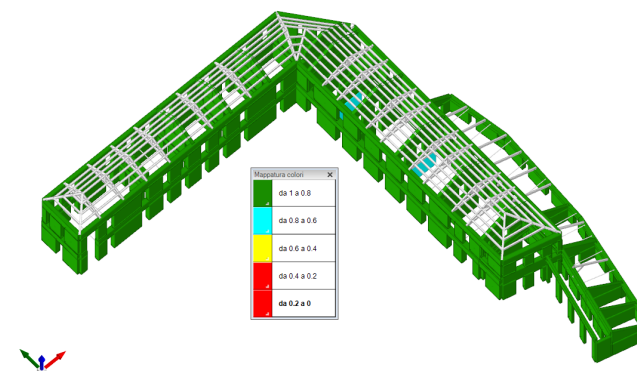
Verifiche statiche degli elementi in muratura
