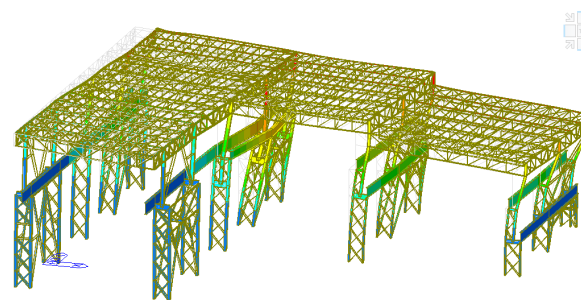
Modello FEM dell'immobile
