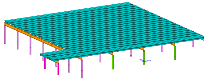
Modello FEM di un corpo del complesso industriale
