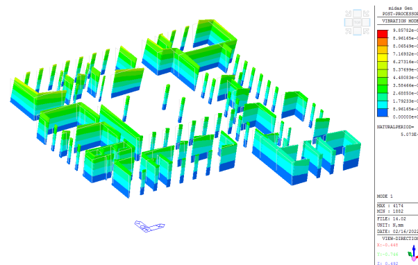
Principale modo di vibrare dell'immobile
