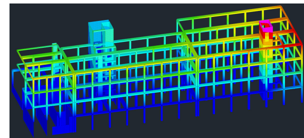
Verifiche strutturali sugli elementi portanti verticali - ala moderna
