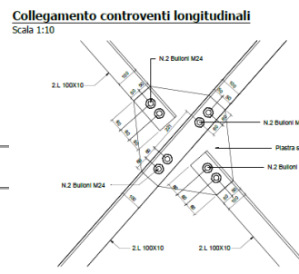
Dettaglio delle connessioni dei controventi
