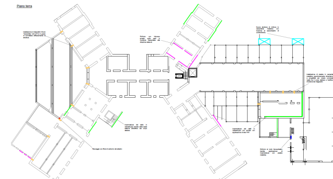
Definizioni degli interventi sul corpo principale
