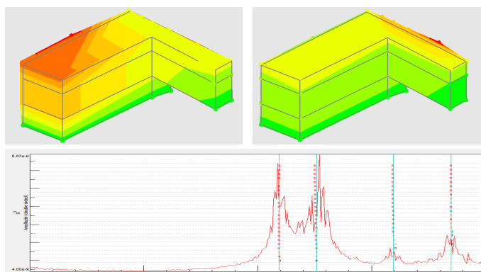
Modi di vibrare ricavati dall'analisi dinamica sperimentale
