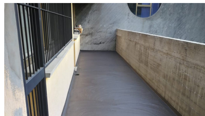
Impermeabilizzazione dei balconi esistenti
