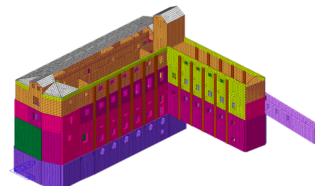
Modello FEM del fabbricato
