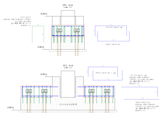
Progetto di consolidamento della fondazione del pilastro
