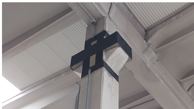
Placcaggio del nodo trave-pilastro
