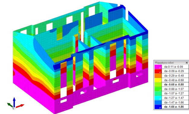
Verifiche degli elementi portanti del fabbricato
