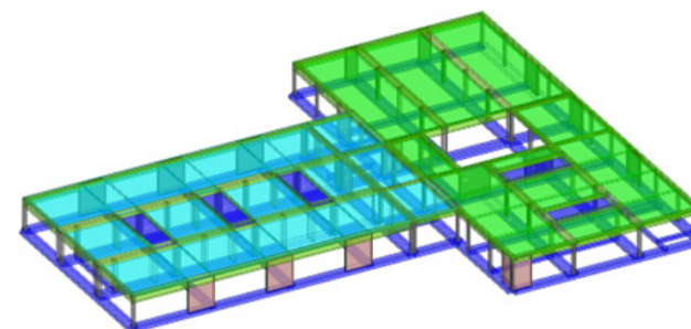
Modello FEM del fabbricato
