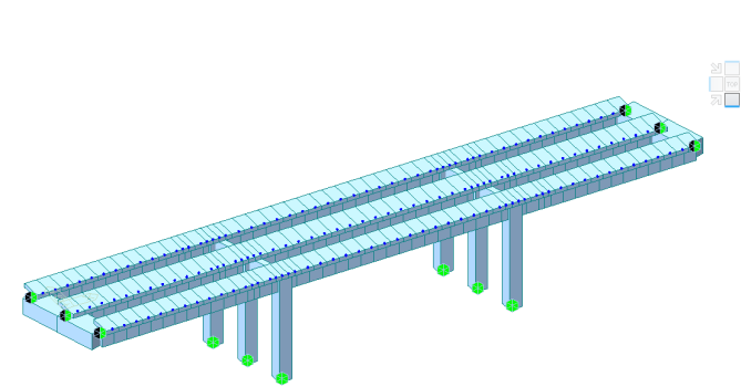
Modello FEM del ponte n.4
