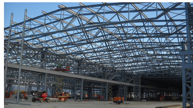
Copertura metallica in travi reticolari
