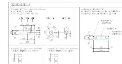
Dettagli di progetto di adeguamento sismico
