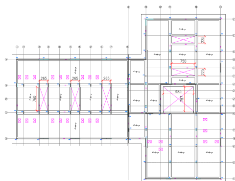
Planimetria con identificazione degli elementi strutturali
