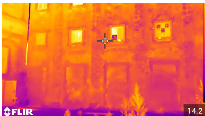
Esecuzione di indagini termografiche
