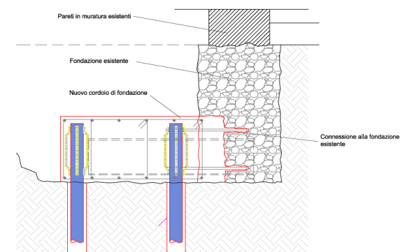
Dettaglio dell'intervento di consolidamento fondazionale
