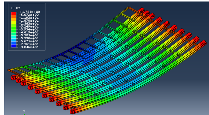
Modello FEM del nuovo ponte per l'analisi delle deformazioni
