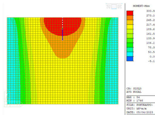
Momento flettente con vincolo di cerniera
