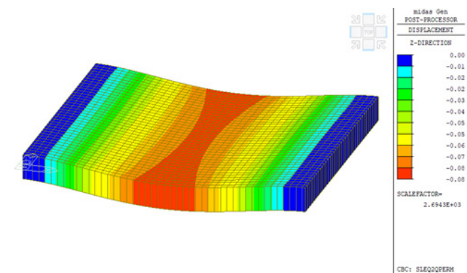
Freccia in combinazione quasi permanente vincolo di incastro
