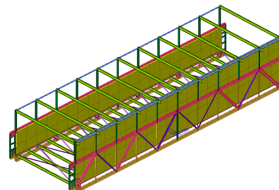
Modello FEM della passerella lato ANAS
