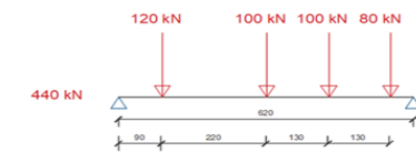
Schema disposizione dei carichi
