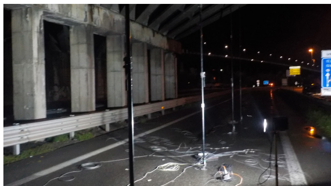
Strumenti di misura posizionati
