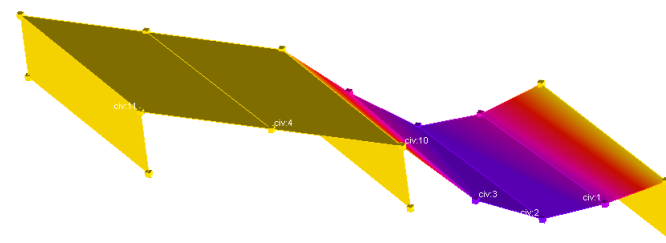
Modo di vibrare principale ottenuto dalla prova dinamica
