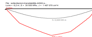
Momento flettente sollecitante - SLU - transitabilità mezzi pesanti
