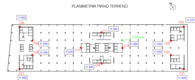
Planimetria delle installazioni
