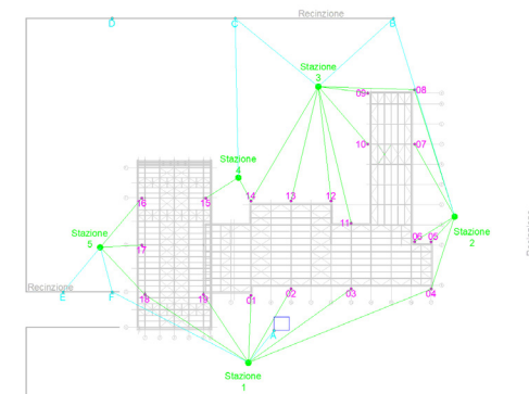
Schema planimetrico rete topografica
