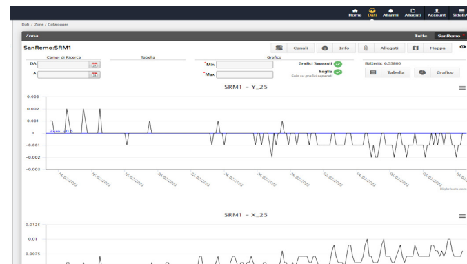
Variazione della verticale inclinometrica nel tempo
