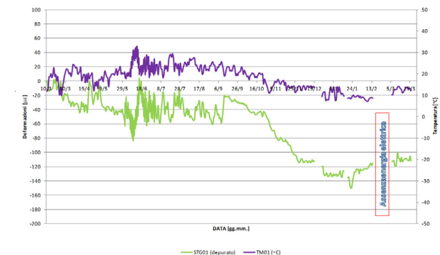
Grafici elaborati dai dati acquisiti
