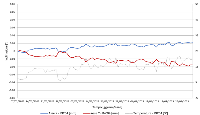
Grafico variazione inclinazione
