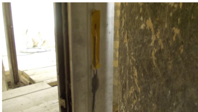
Estensimetro su profilato in acciaio
