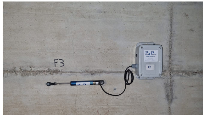
Installazione tipo fessurimetro
