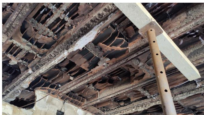
Analisi visiva sui solai
