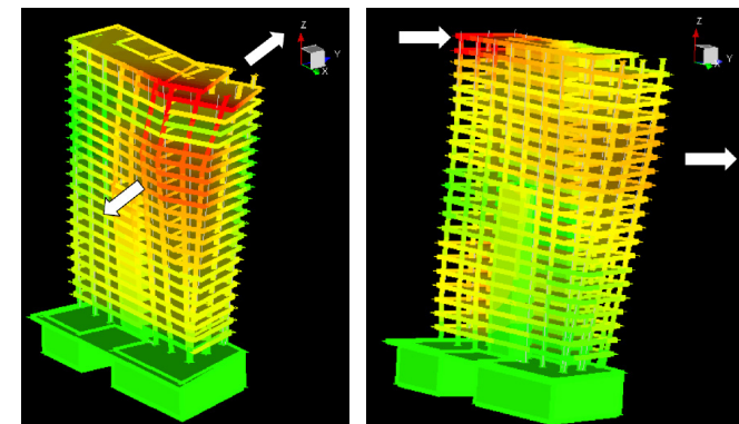
Risultati del monitoraggio dinamico in corso d'opera
