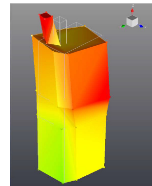
Modi principali di vibrare della torre
