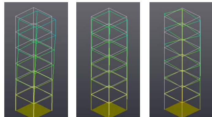
Modi sperimentali di vibrare della struttura
