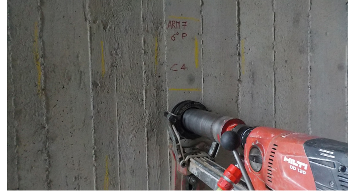
Esecuzione di carotaggio per prova di compressione
