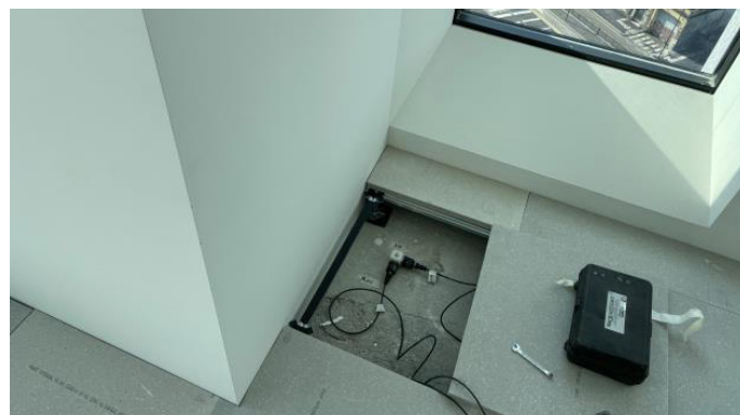
Posa di accelerometro per prova dinamica
