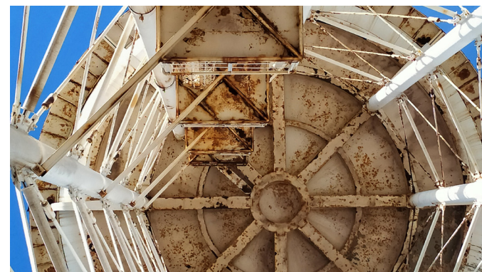
Rilievo del degrado dell'intradosso del serbatoio
