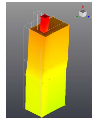
Modi principali di vibrare della torre
